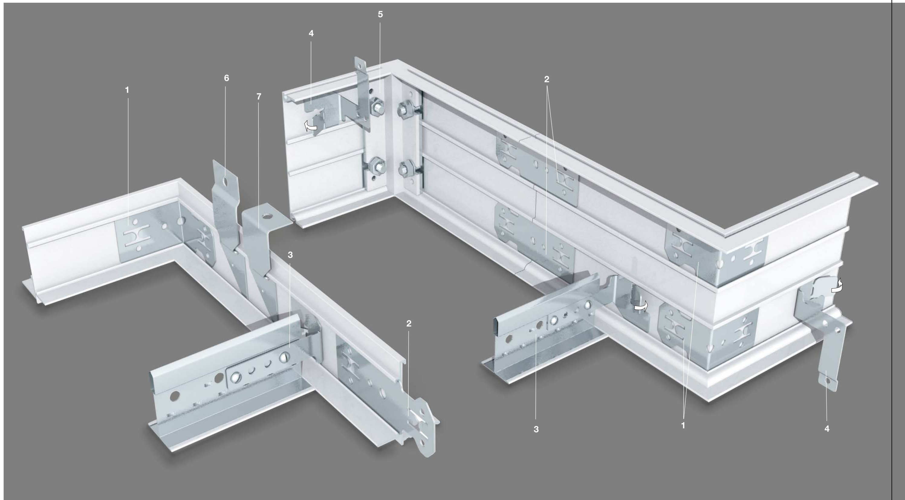
1 Clip d'angle universel Axiom Clip d'angolo universale Axiom BPA 340 G
